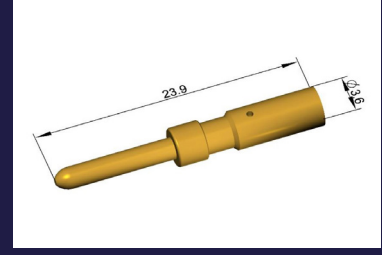
Crimpkontakte
