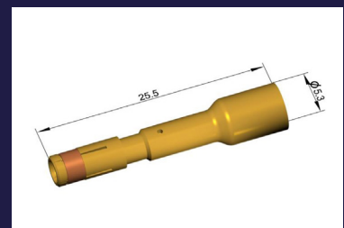
Crimpkontakte
